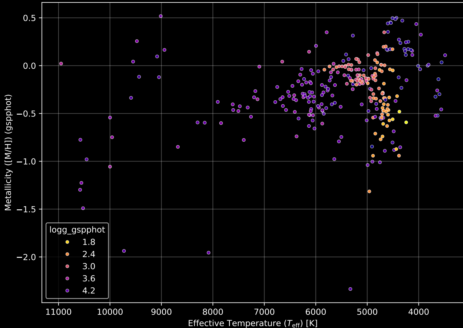
APOGEE DR17 Field: [ORIONOB1AB-F] Stellar Population Parameters (n= 293)
